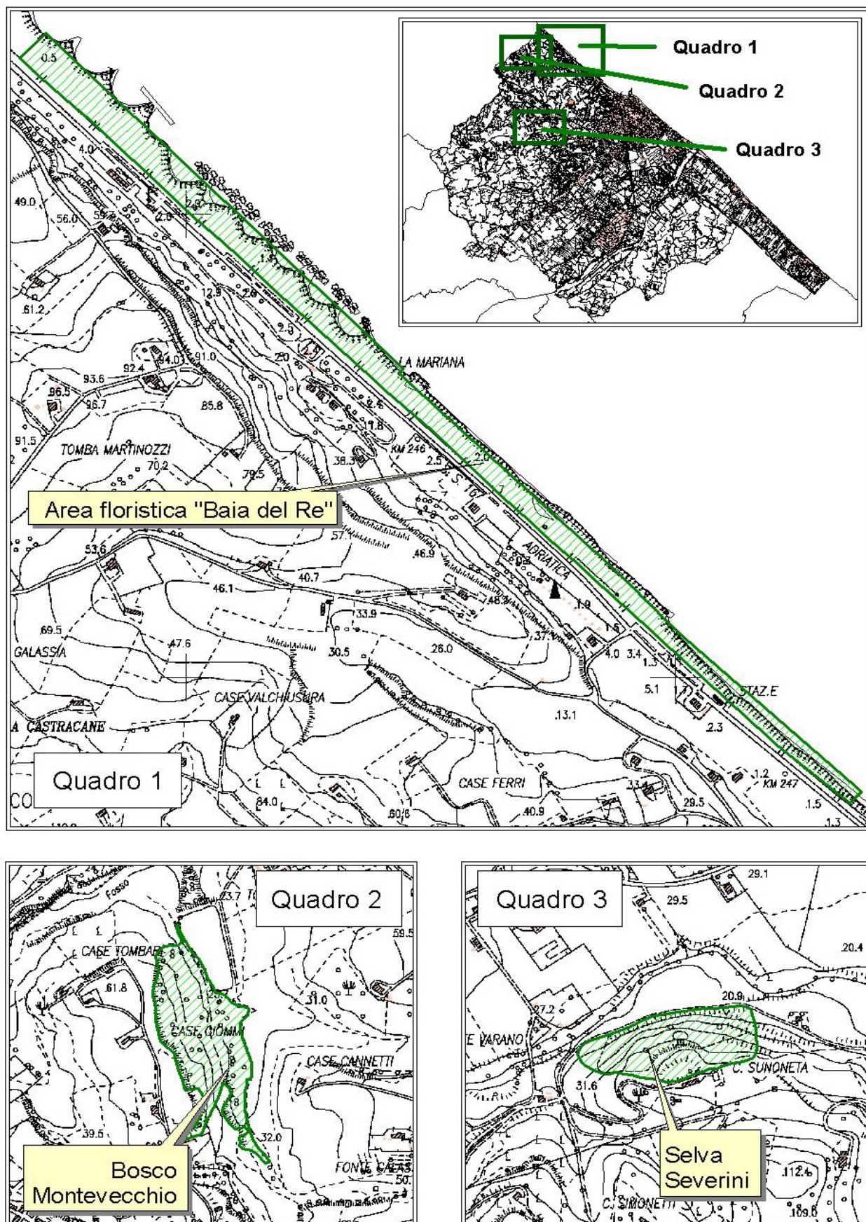
Fig. 3.4. Mappatura delle aree floristiche protette. Su base cartografica di proprietà della Regione Marche – uff. Cartografia e Informazioni Territoriali
