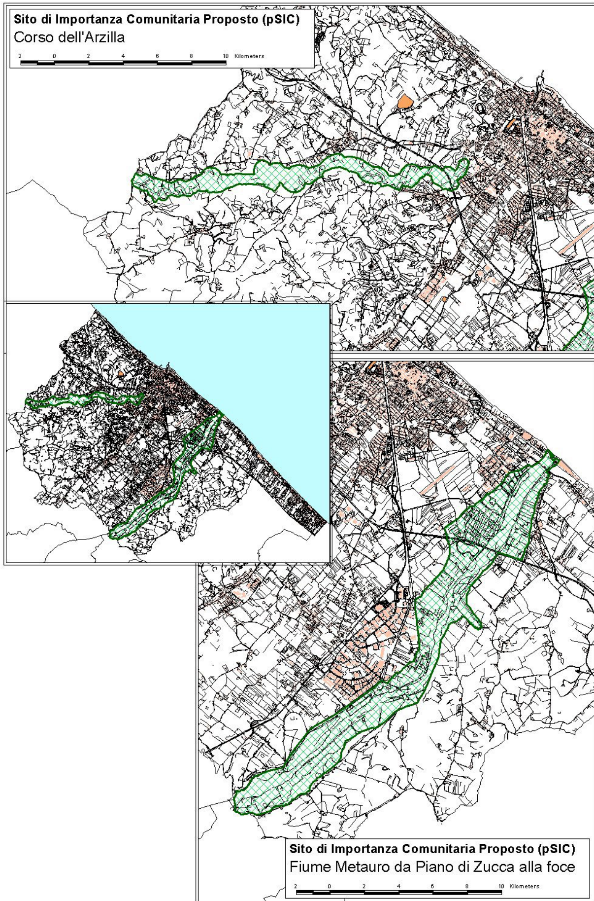
Figura 3.6. Siti di Importanza Comunitaria (pSIC)
