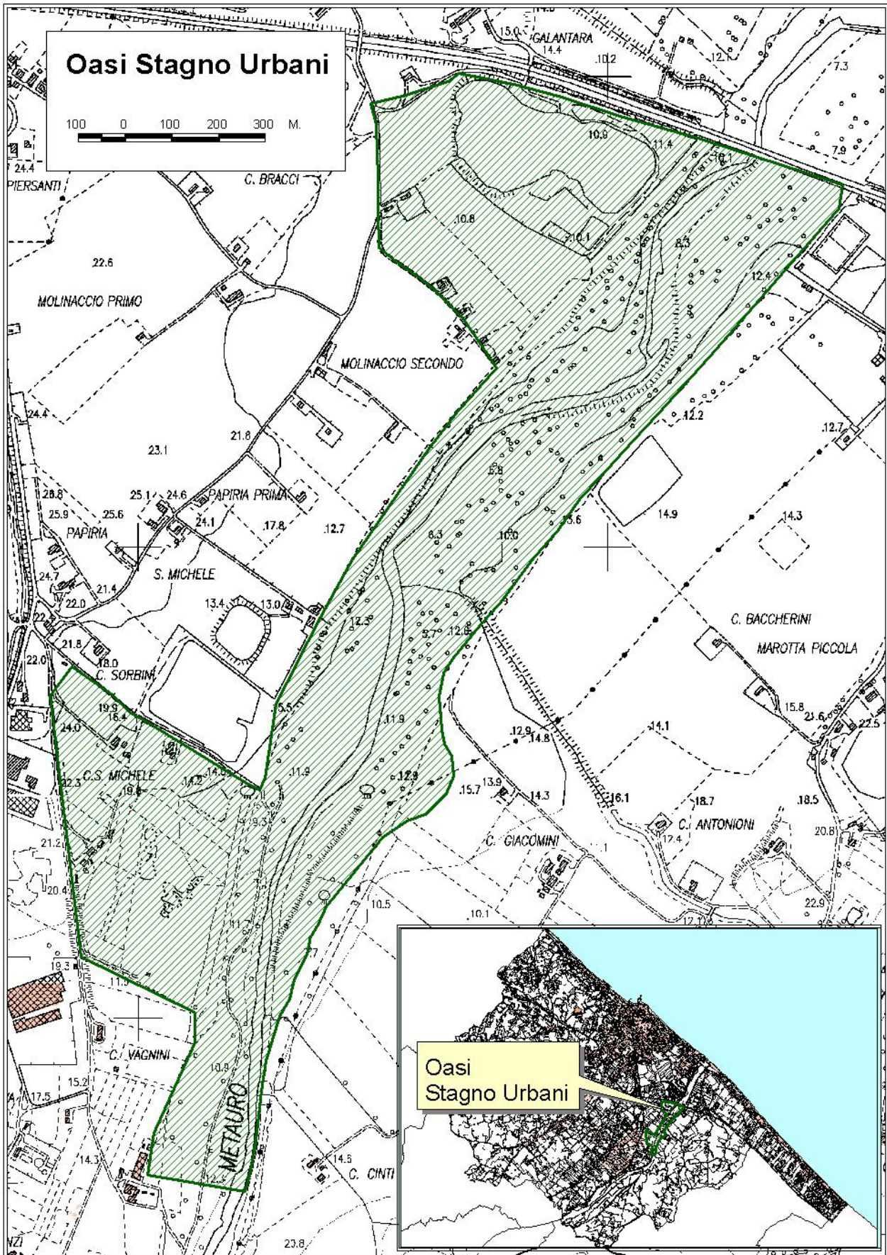
Fig. 3.5. Mappatura Oasi Stagno Urbani.
