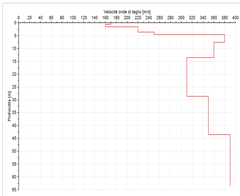
Profilo delle velocità delle onde di taglio.
