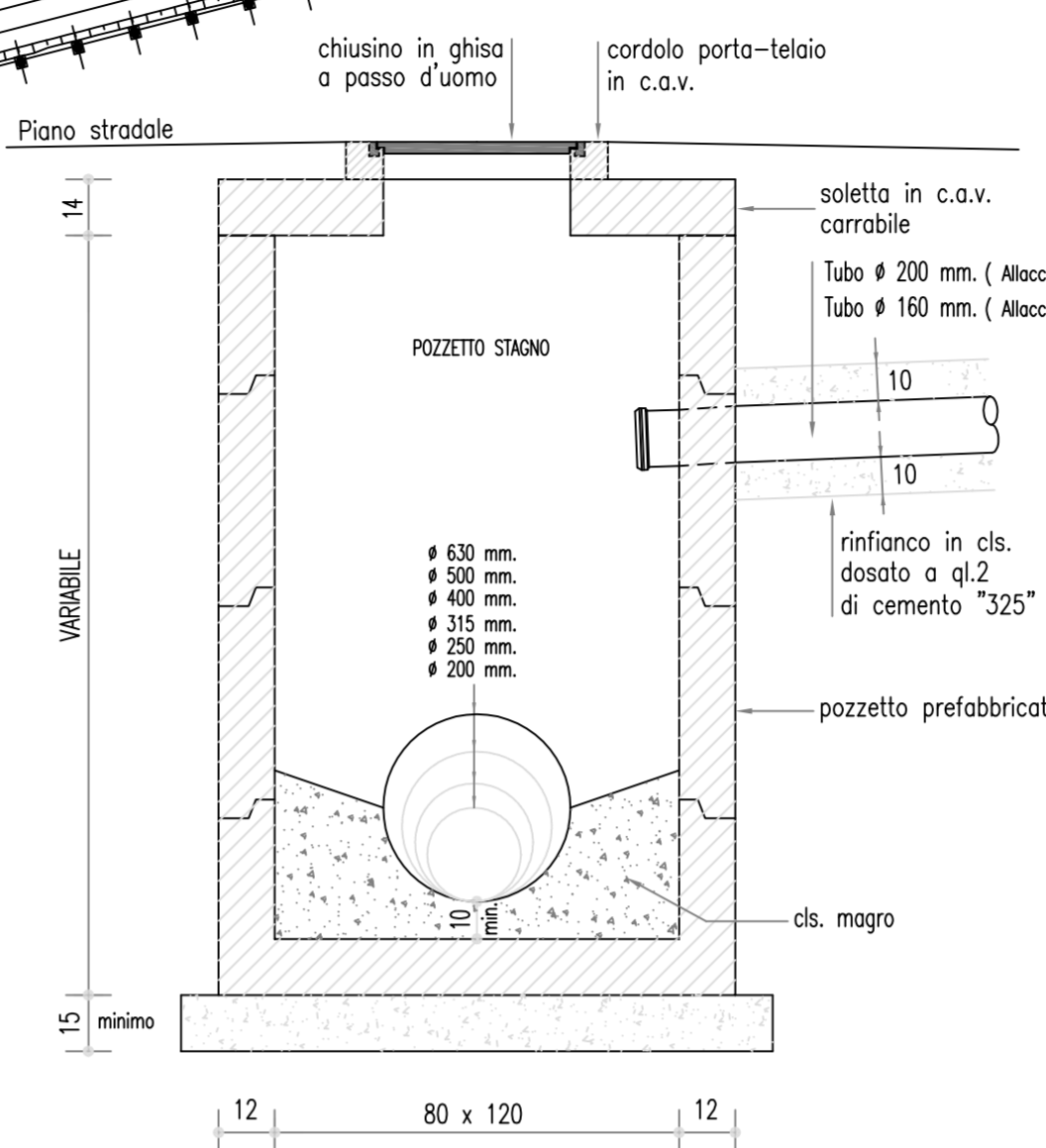
PARTICOLARE TIPICO POZZETTO D'ISPEZIONE Scala 1:20
