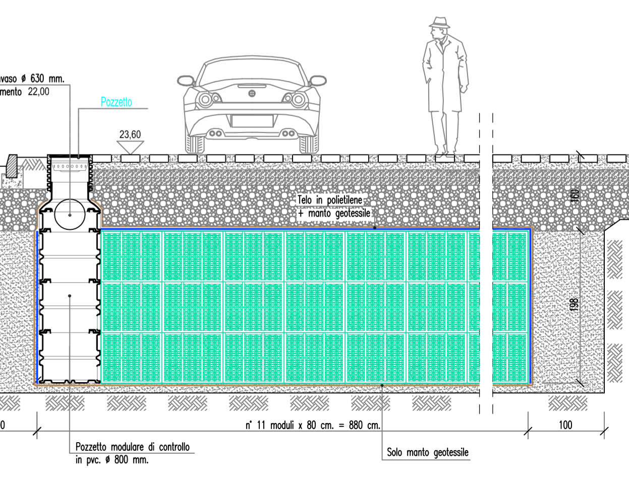
SEZIONE X-X scala 1:50
