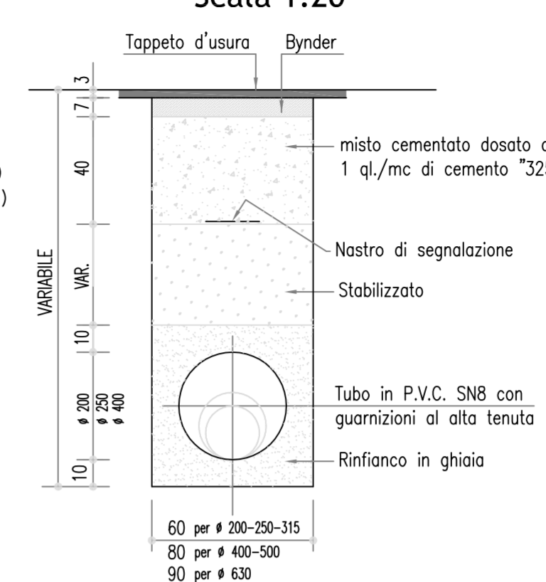
PARTICOLARE TIPICO SEZIONE DI SCAVO Scala 1:20
