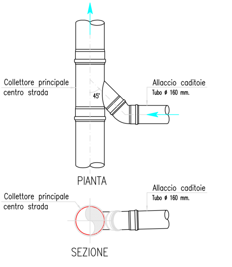
PARTICOLARE TIPICO ALLACCIO CADITOIE ed UTENZE Scala 1:20
