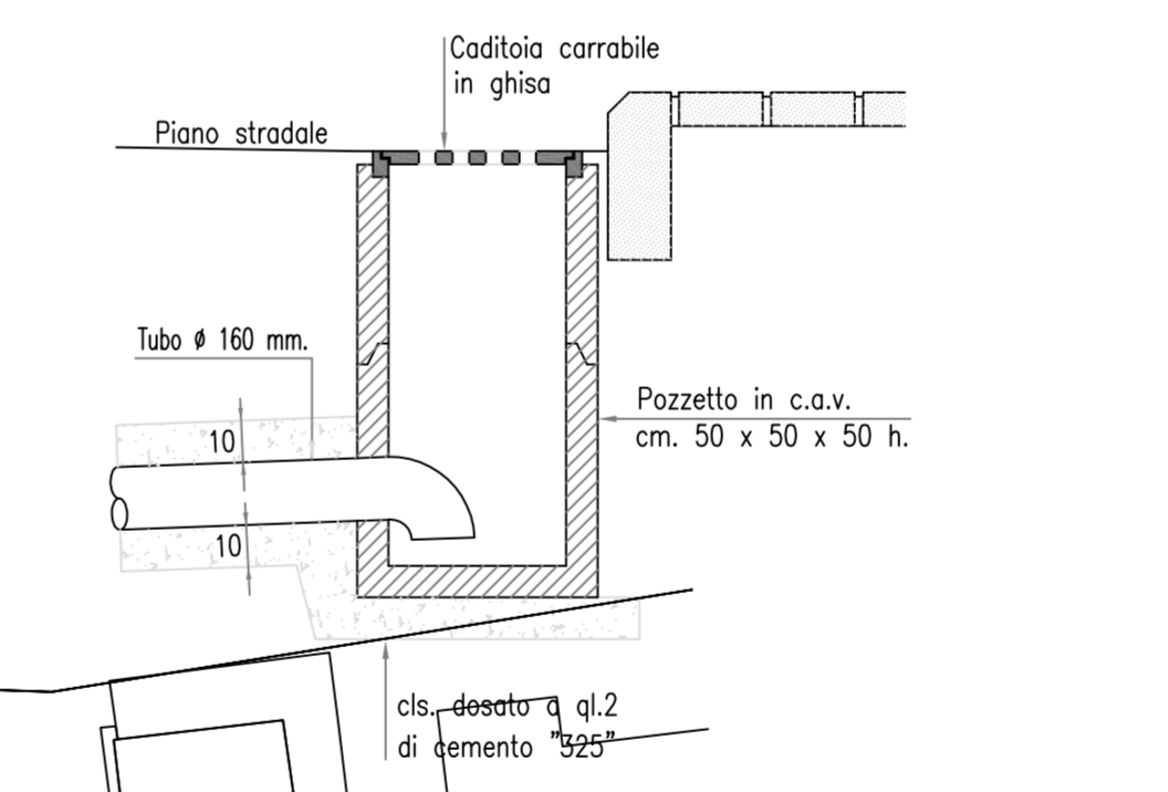
SEZIONE Y-Y scala 1:50
