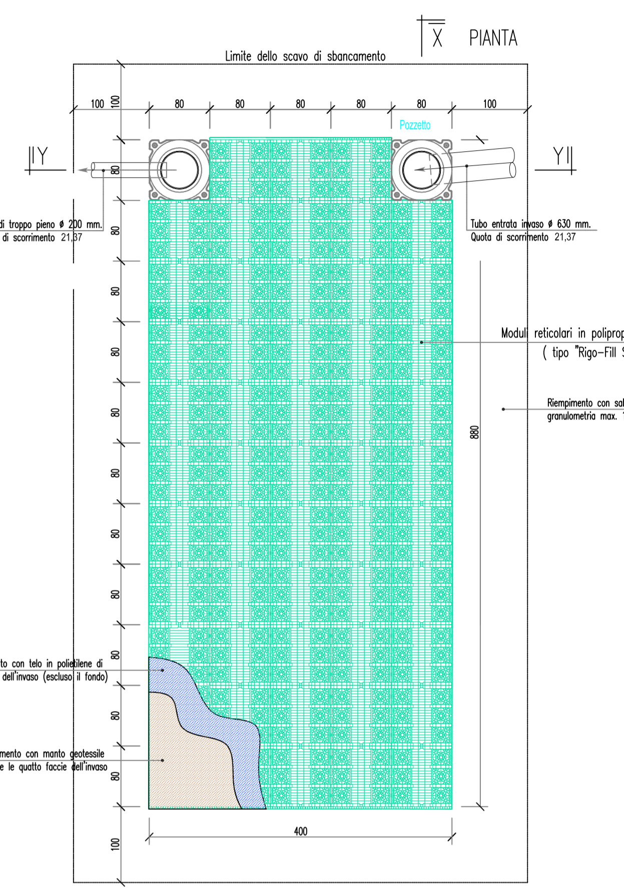
INVASO DI LAMINAZIONE E DISPERSIONE "A" (Mc. 70) Scala 1:50
